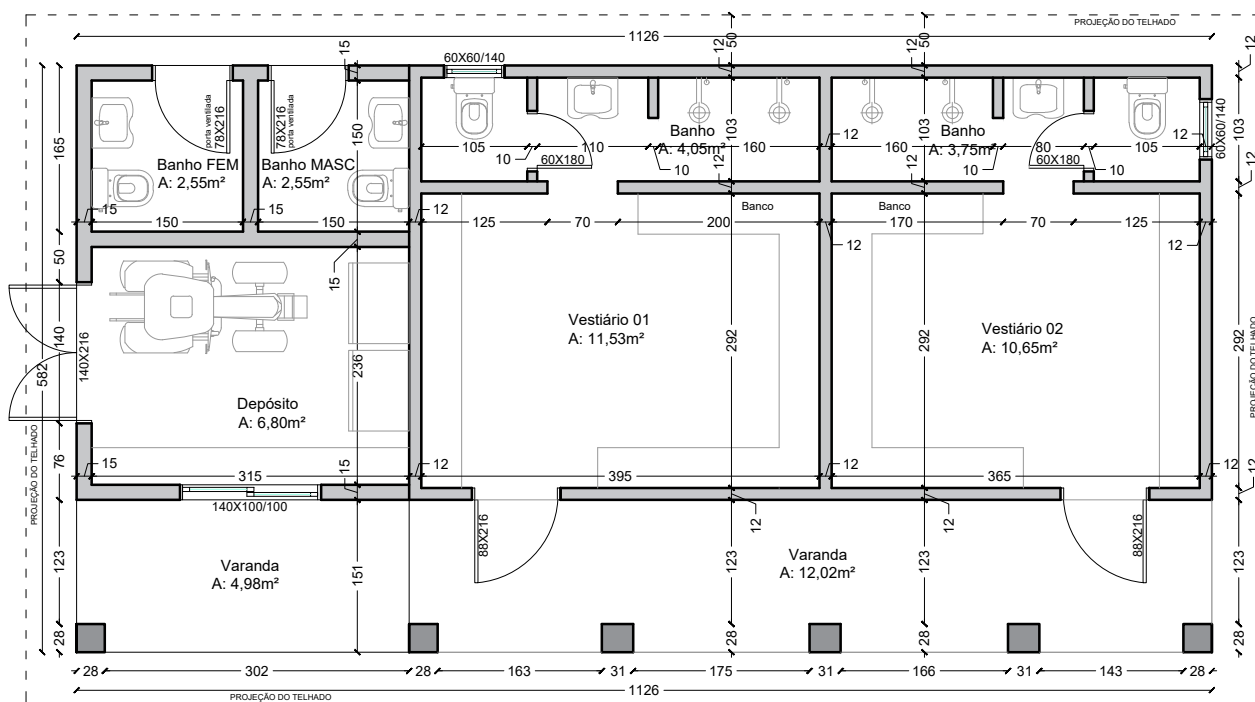
PLANTA BAIXA DA PROPOSTA ÁREA: 65,50M 2 ESC: 1/75
