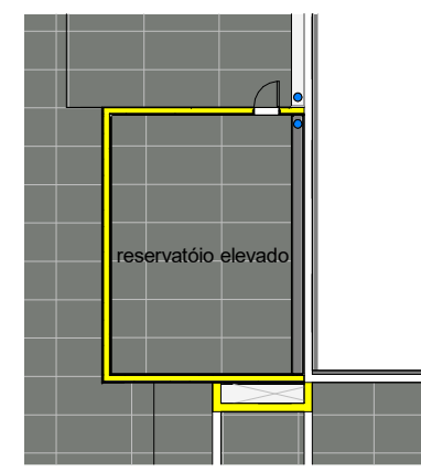
3 RESERVATÓRIO ESCALA 1 : 200
