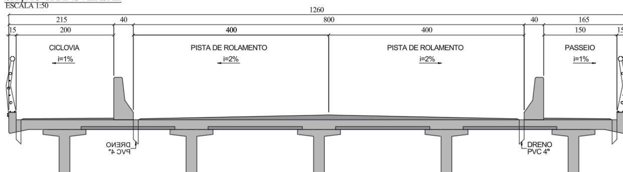
Figura 02 – Seção transversal com duas pistas de rolamento de 4,00 m protegidas por barreira tipo New Jersey e laterais sendo uma com passeio simples de 1,50 m protegido por guarda-corpo metálico e outra com ciclovia de 2,00 m protegida por guarda-corpo metálico.
