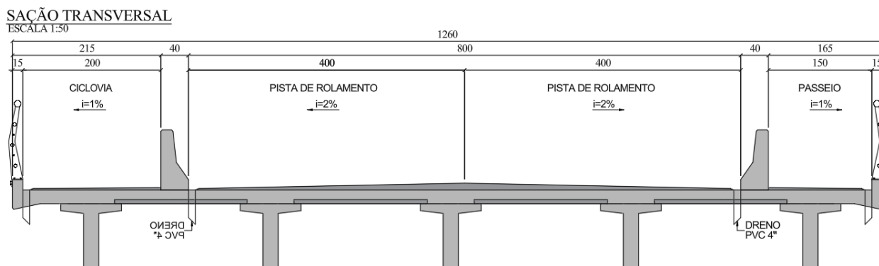
Figura 02 – Seção transversal com duas pistas de rolamento de 4,00 m protegidas por barreira tipo New Jersey e laterais sendo uma com passeio simples de 1,50 m protegido por guarda-corpo metálico e outra com ciclovia de 2,00 m protegida por guarda-corpo metálico.
