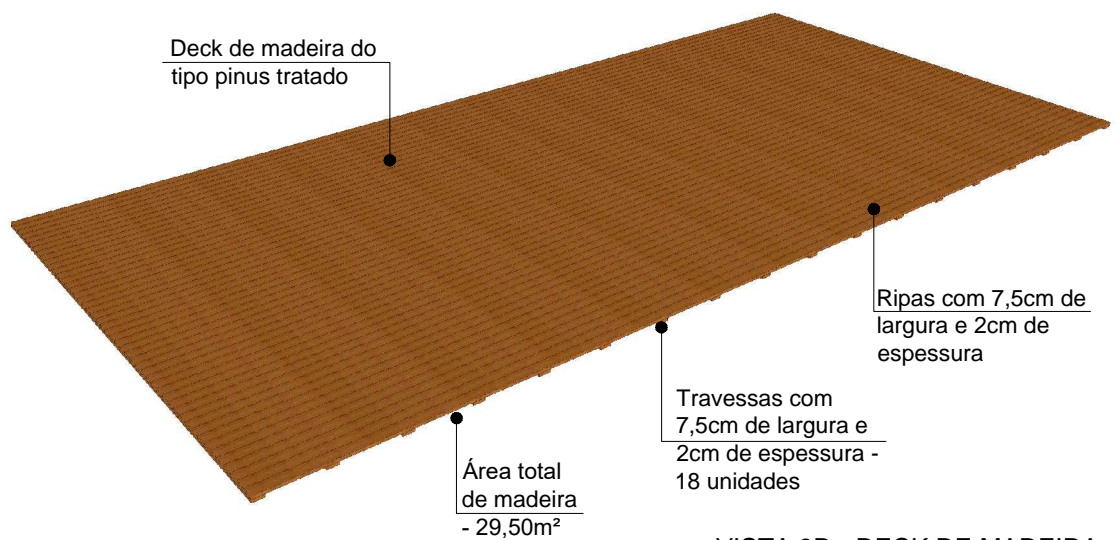
VISTA 3D - DECK DE MADEIRA Escala: 1/50
