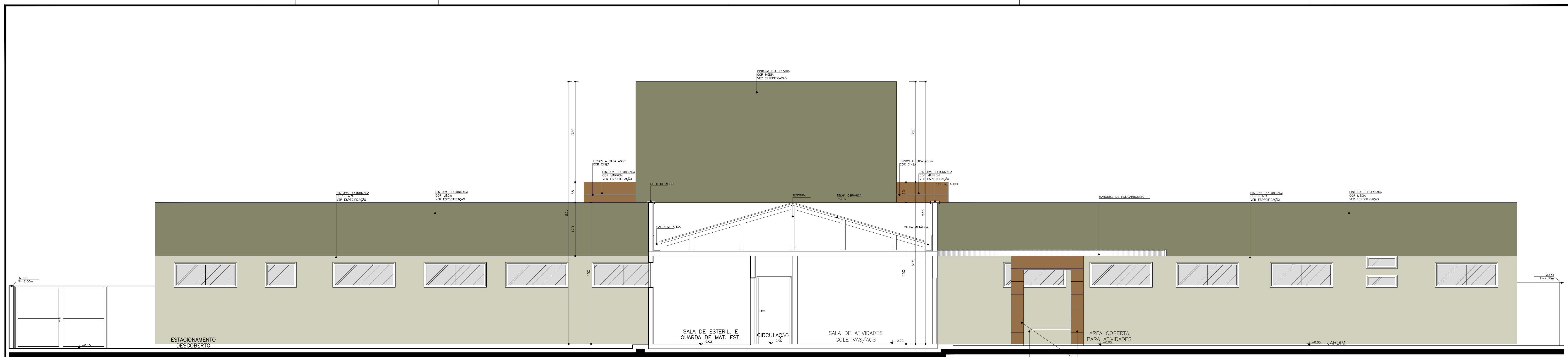
Corte DD' Esc.: 1:50
