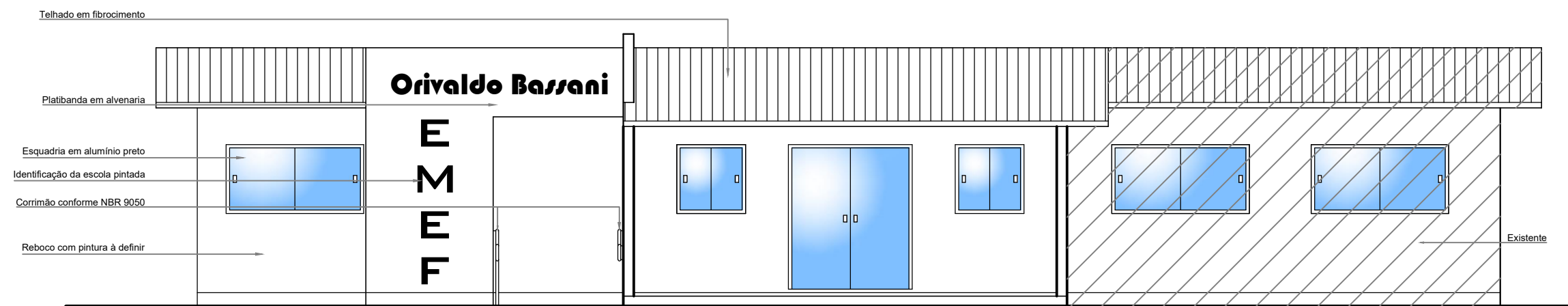
FACHADA Escala 1:75
