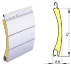
Palhetas de persianas
