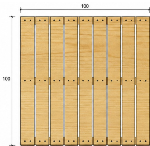
Figura 1 - Imagens ilustrativas representando a montagem do deck modular conforme especificações.
