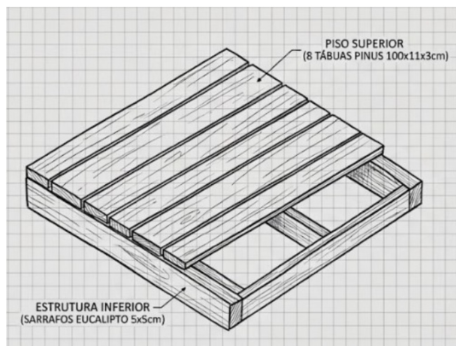
Figura 1 - Imagens ilustrativas representando a montagem do deck modular conforme especificações.
