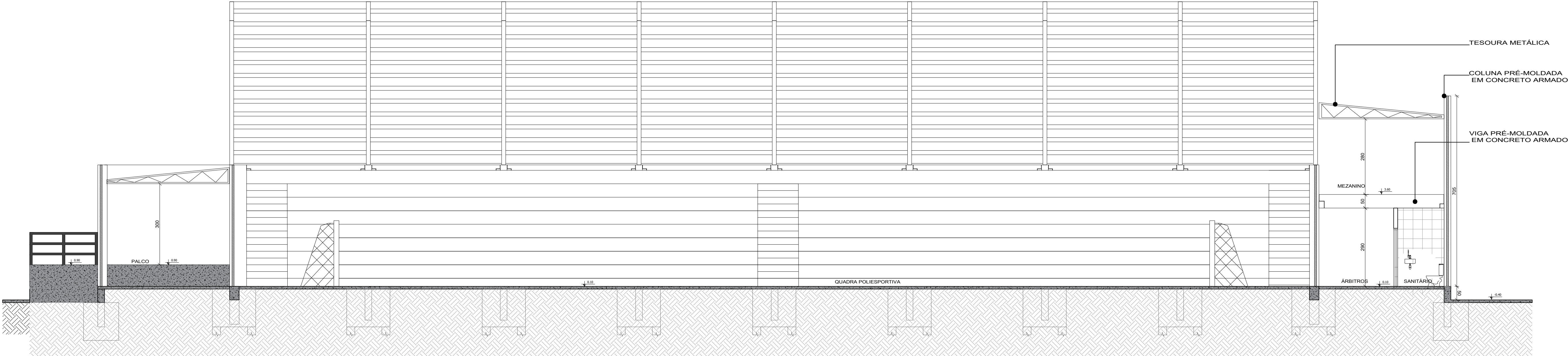
Corte AA'
