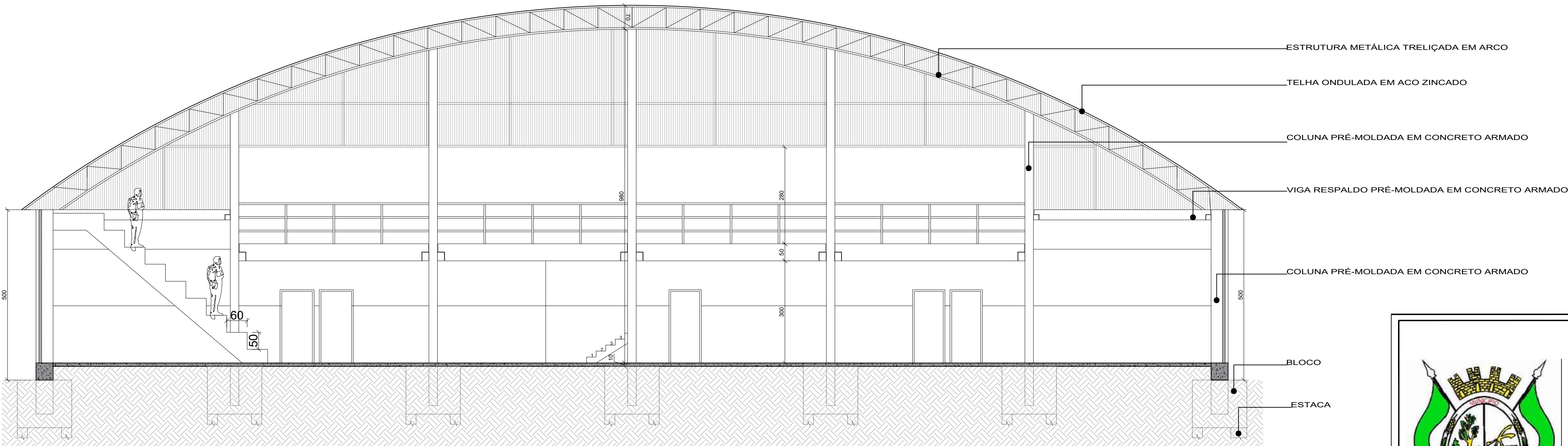
Corte CC'
