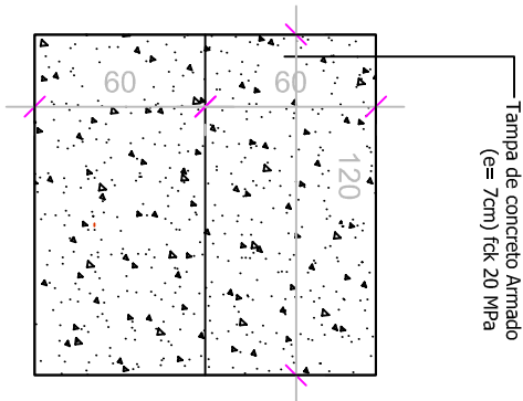
PLANTA BAIXA - TAMPA
