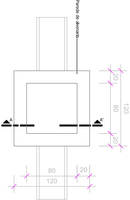
PLANTA BAIXA
