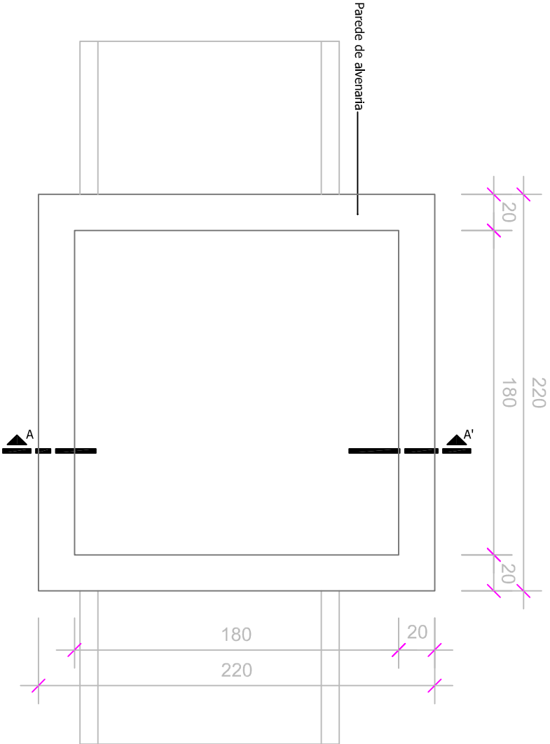
PLANTA BAIXA
