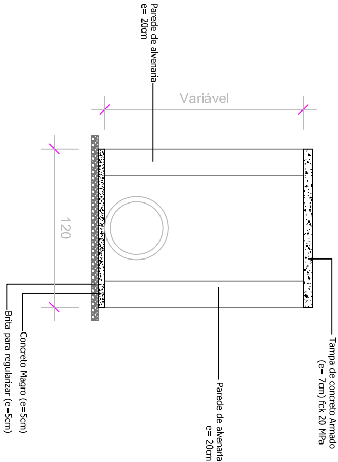
CORTE A-A'
