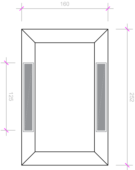
PLANTA BAIXA
