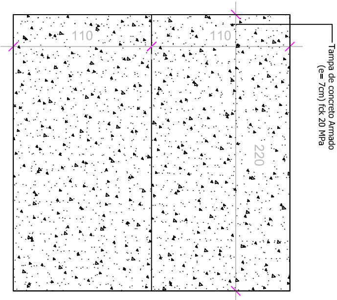
PLANTA BAIXA - TAMPA
