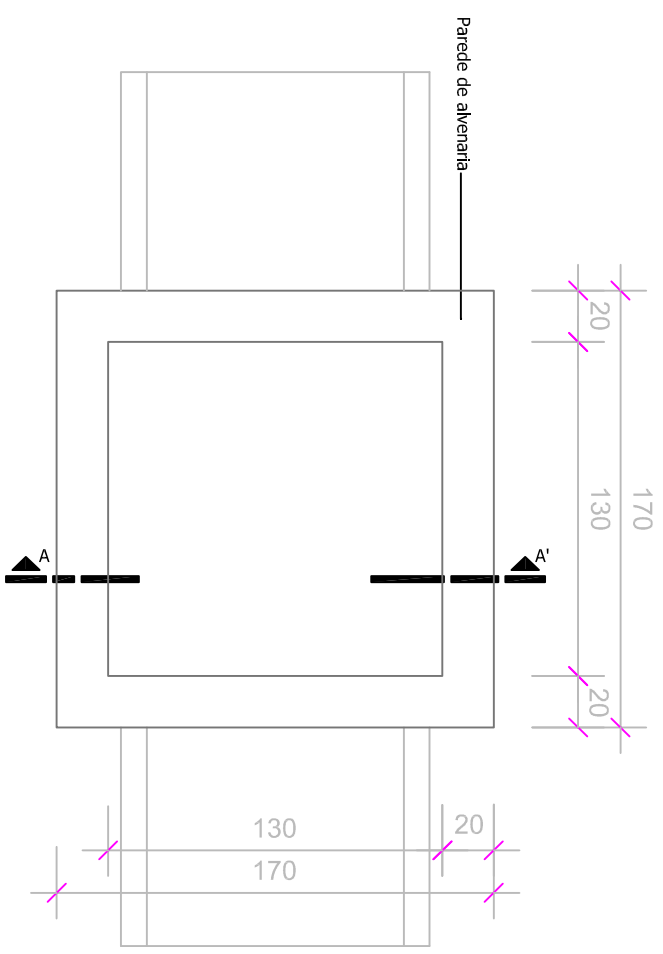
PLANTA BAIXA
