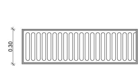
Det. ES-PL-01- Grelha ESC.1/20
