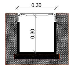
Det. ES-PL-01- Canaleta pluvial ESC.1/20
