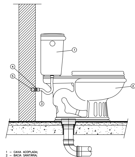
INSTALAÇÃO DO VASO SANITÁRIO COM CAIXA ACOPLADA
