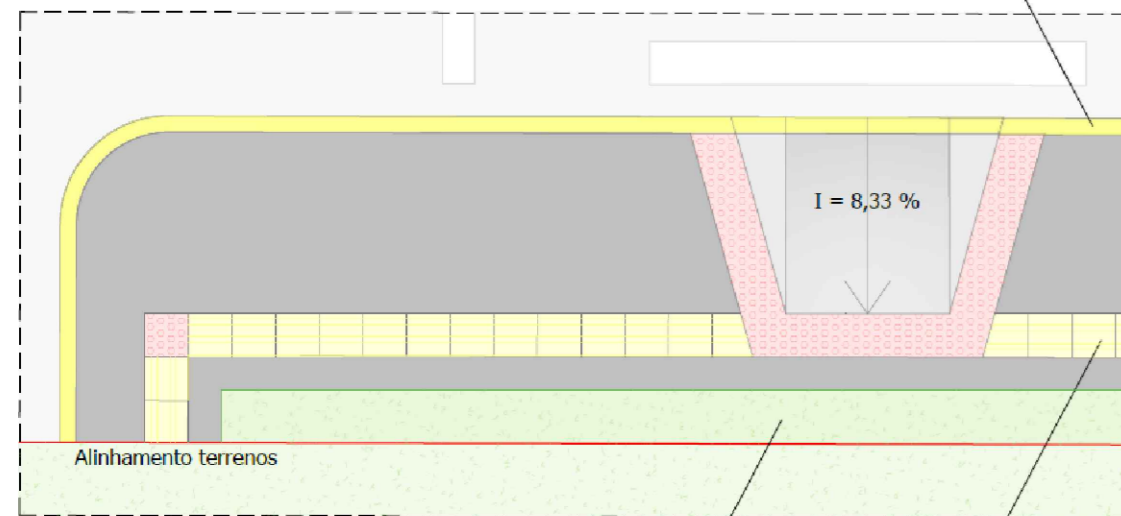
DETALHE 01.1 (S/ escala) Canteiro de grama 50cm Piso podotátil 40x40cm
