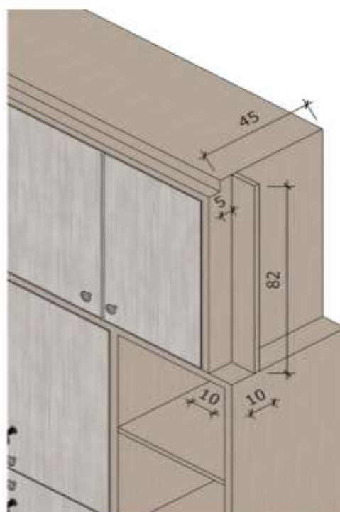
Detalhe devido trilho da cortina existente
