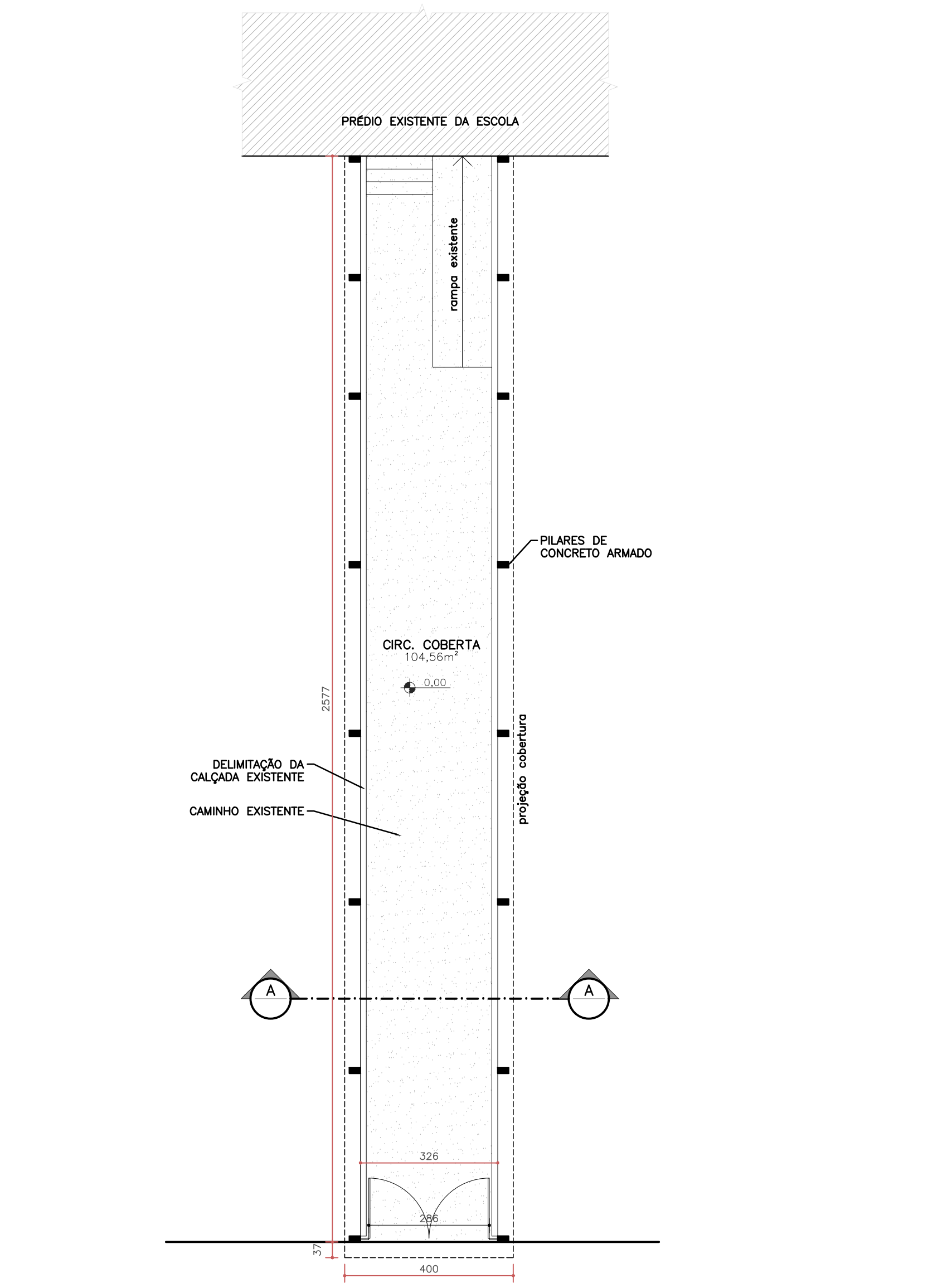
PLANTA BAIXA TERREO ESC. 1:100
