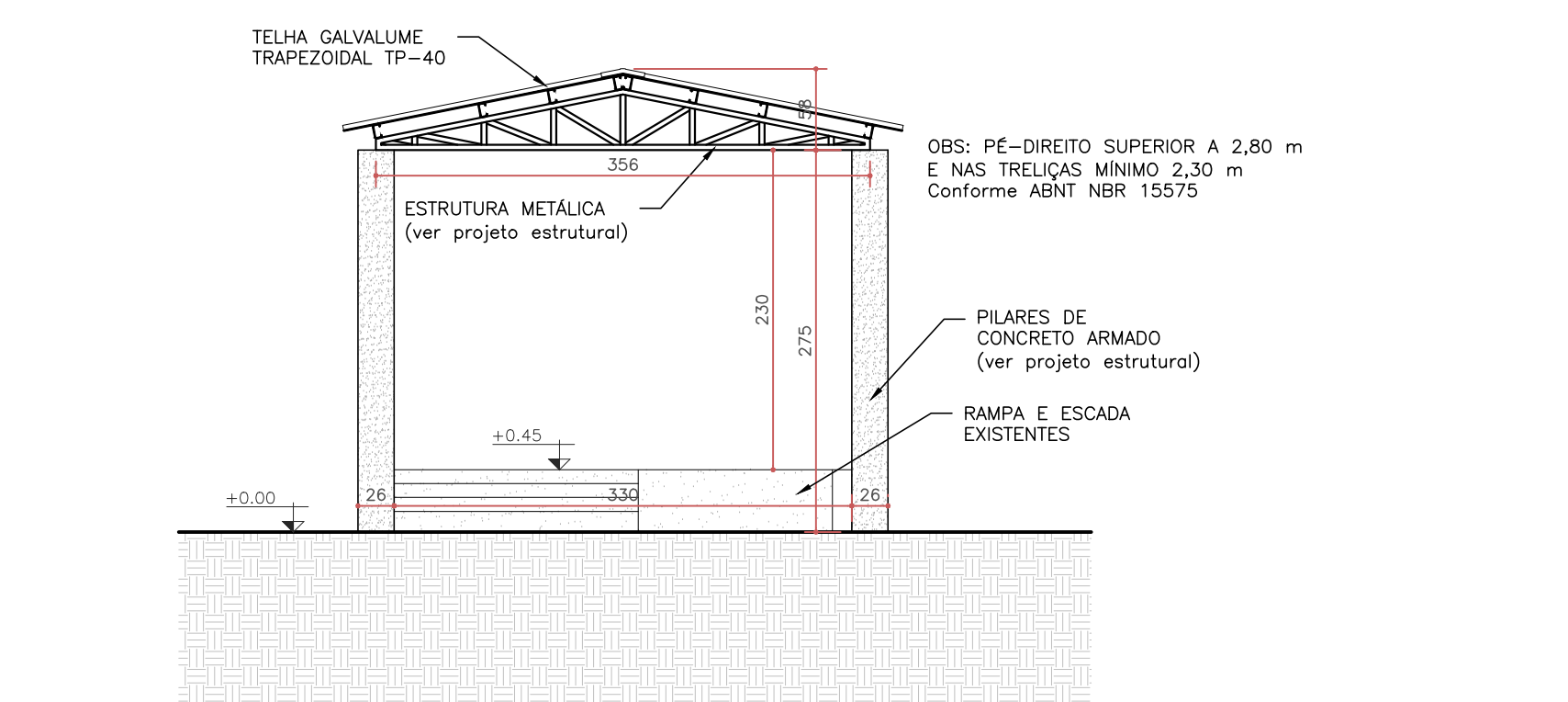
CORTE A ESC. 1:50
