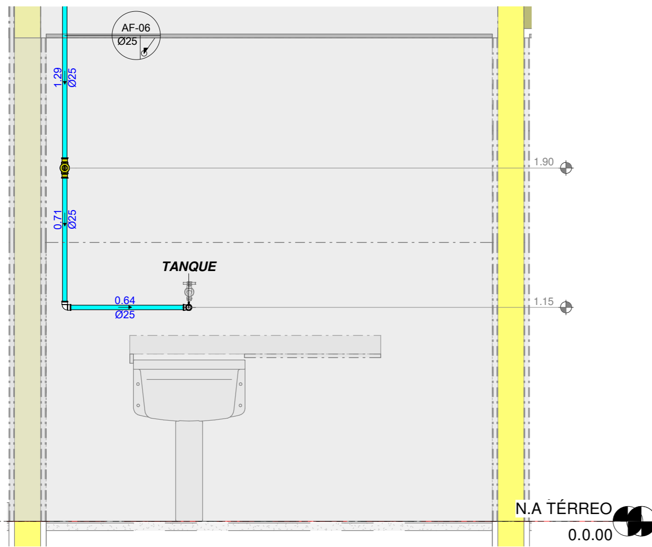
LAVANDERIA - CORTE 1 : 20
