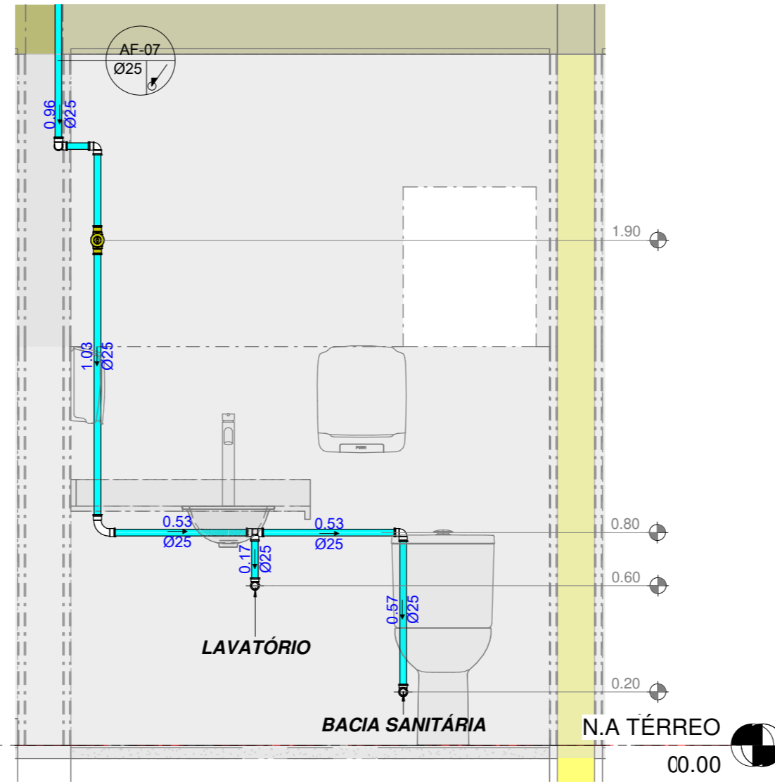
LAVABO - CORTE 1 : 20
