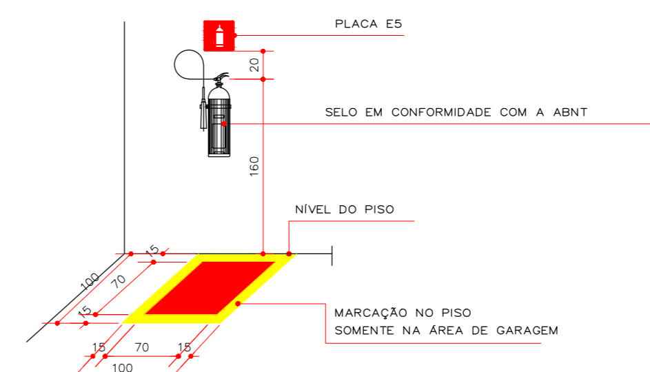
EXTINTOR - DETALHE ESCALA 1:50
