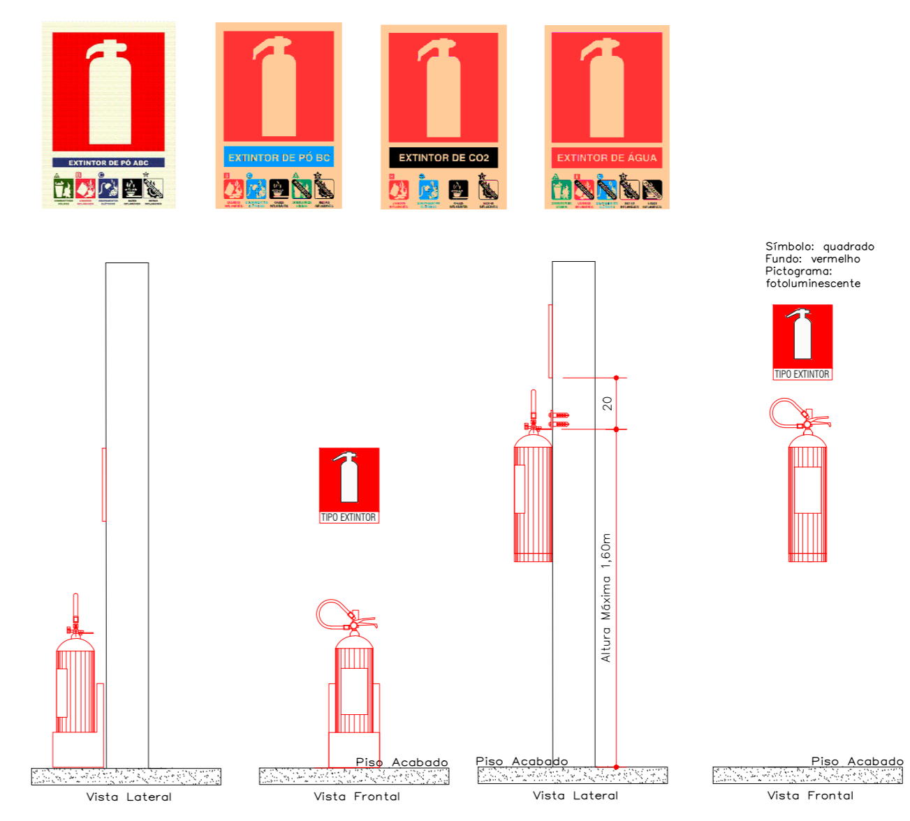
DETALHE - EXTINTORES ESCALA 1:25
