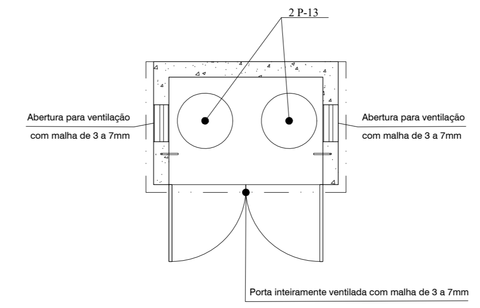
PLANTA BAIXA DETALHE - CENTRAL DE GLP ESCALA 1:25
