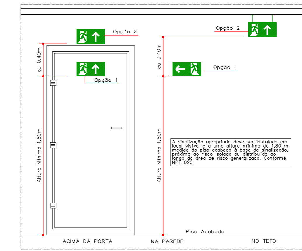
DETALHE - INSTALAÇÃO PLACA ESCALA 1:25
