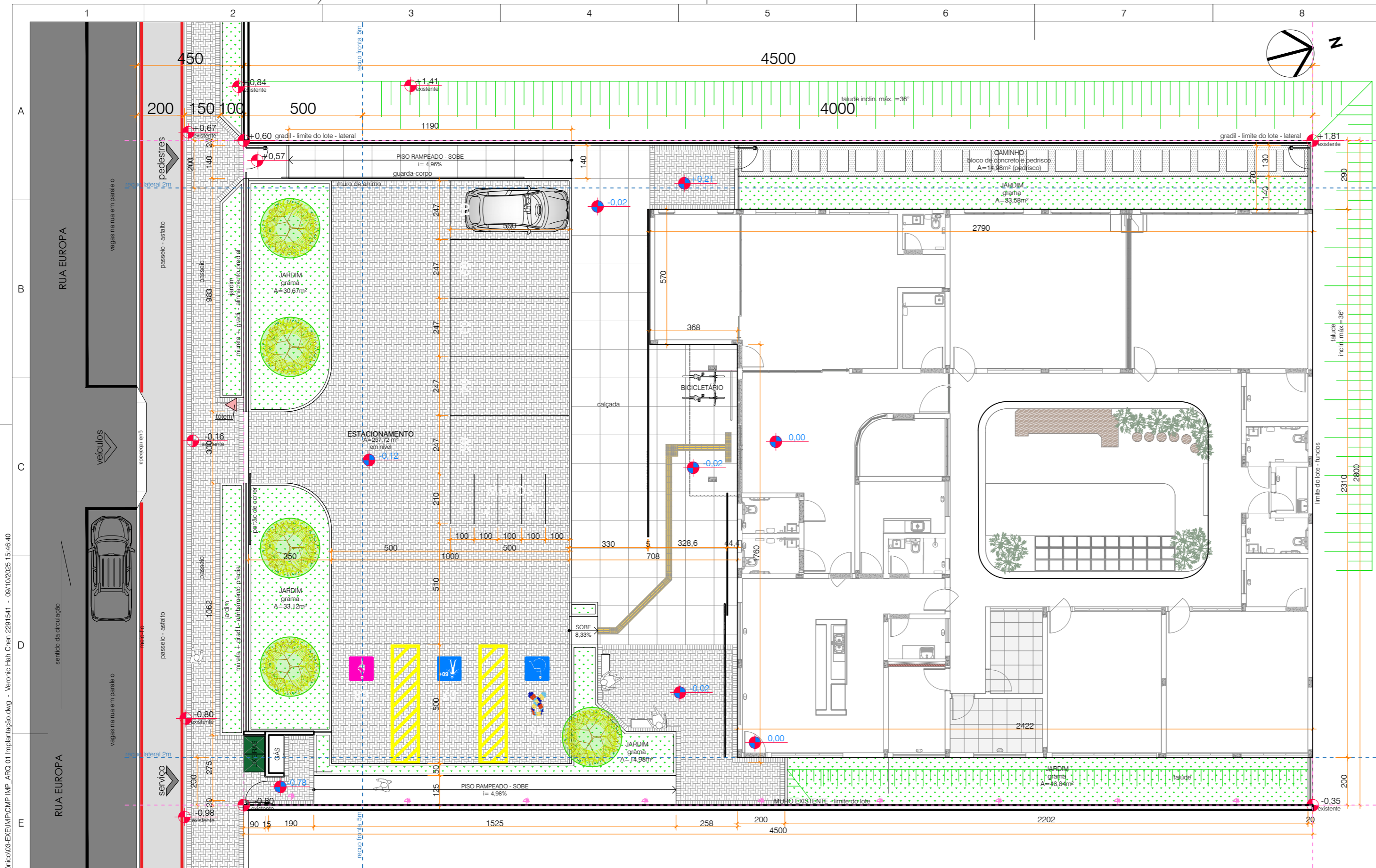
IMPLANTAÇÃO esc 1/150
