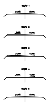
SUPERELEVÇÃO DE CURVA PARA A DIREITA ESCALA 5/2
