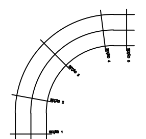
SUPERELEVÇÃO DE CURVA PARA A DIREITA ESCALA 5/2
