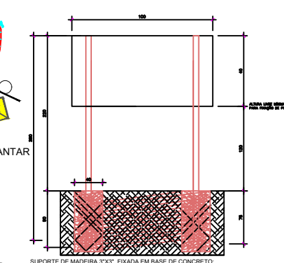
SUPORTE PARA PLACAS DE SINALIZAÇÃO - INDICAÇÃO
