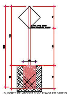
SUPORTE PARA PLACAS DE SINALIZAÇÃO
