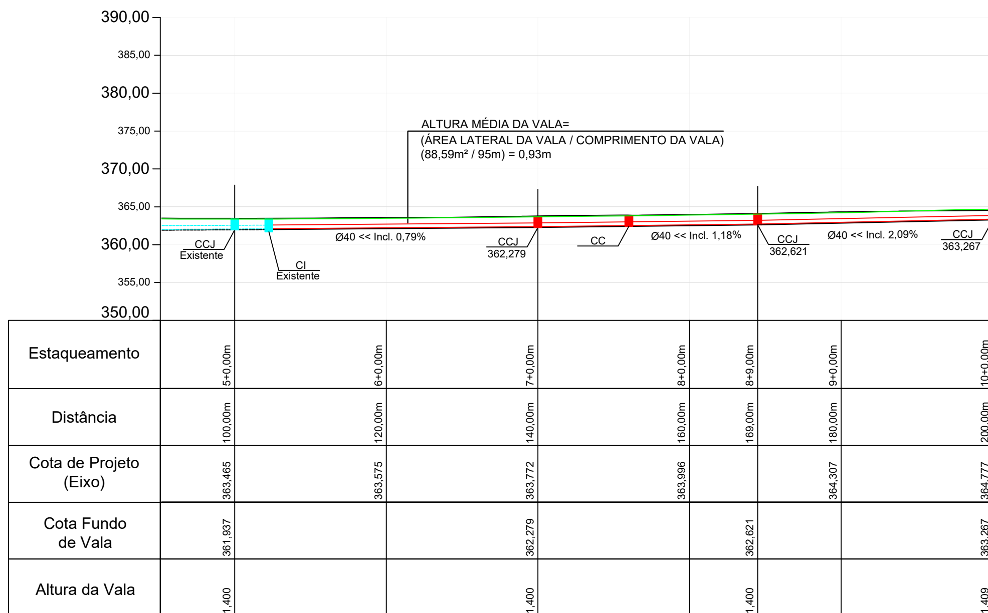
Fundo de Vala - Lado Esquerdo Escala: 1/500
