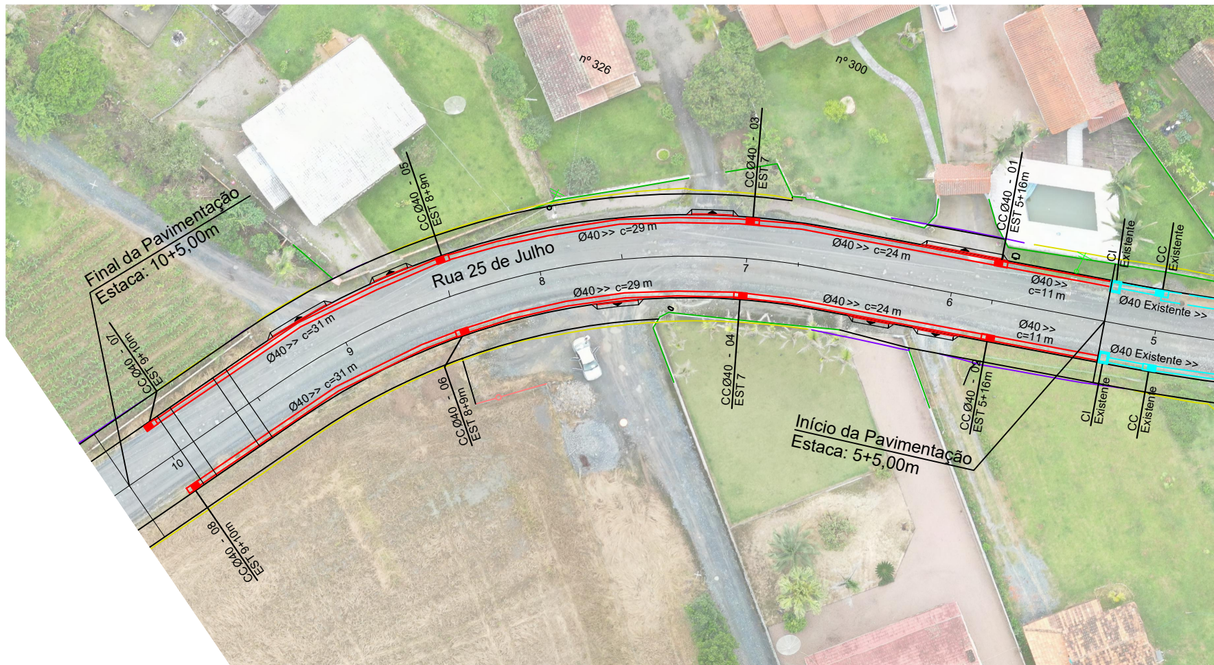
PROJETO DRENAGEM ESC 1/500
