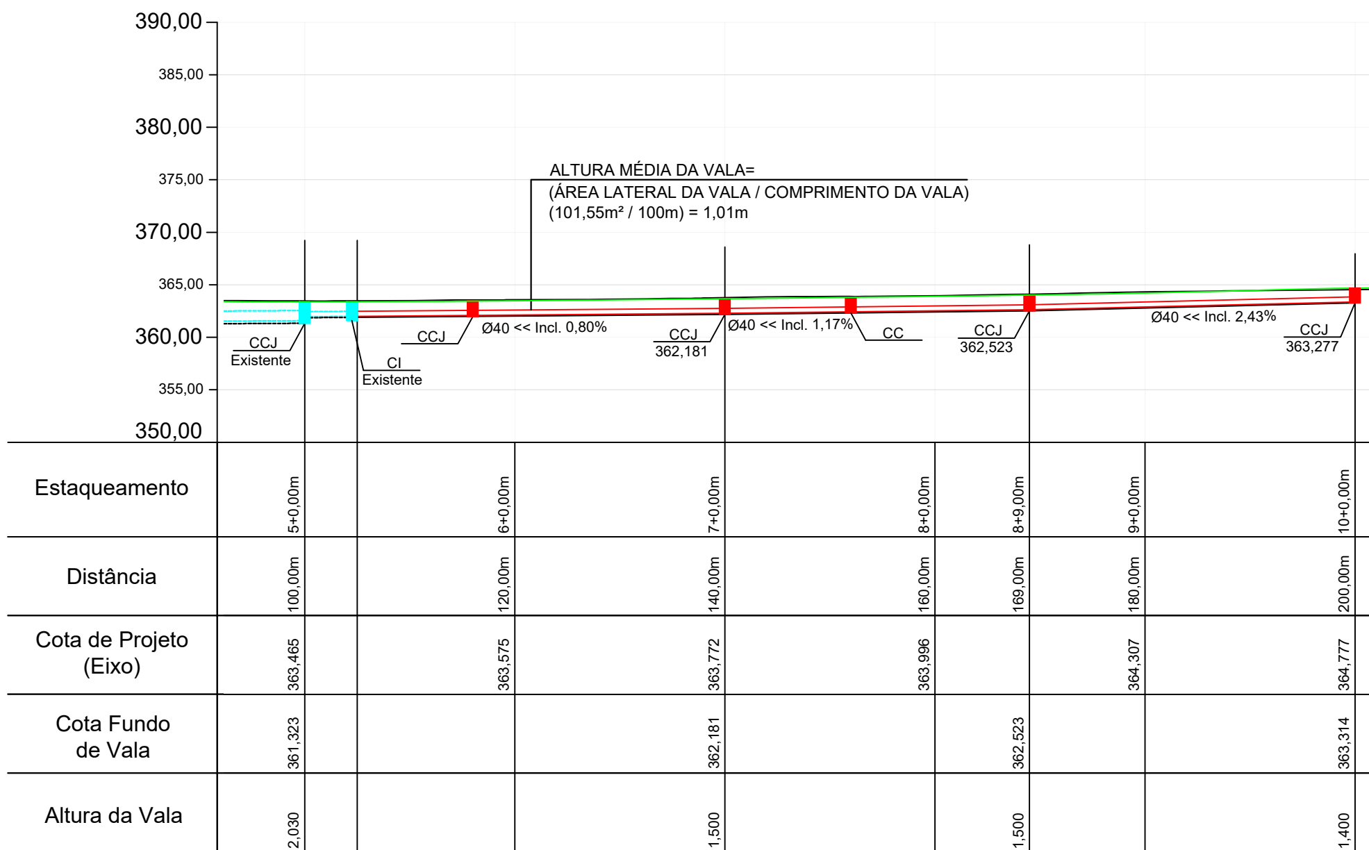
Fundo de Vala - Lado Direito Escala: 1/500
