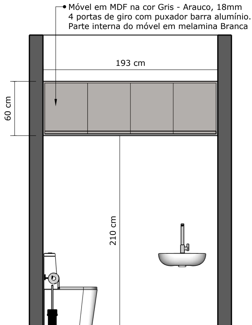
VISTA A
