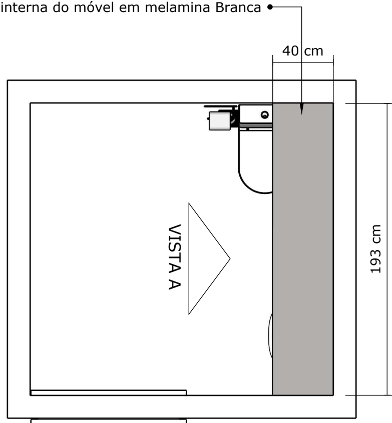
PLANTA BAIXA
