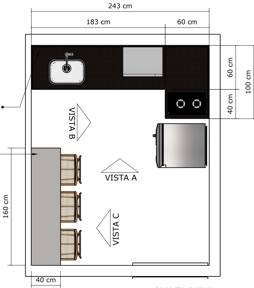
PLANTA BAIXA
