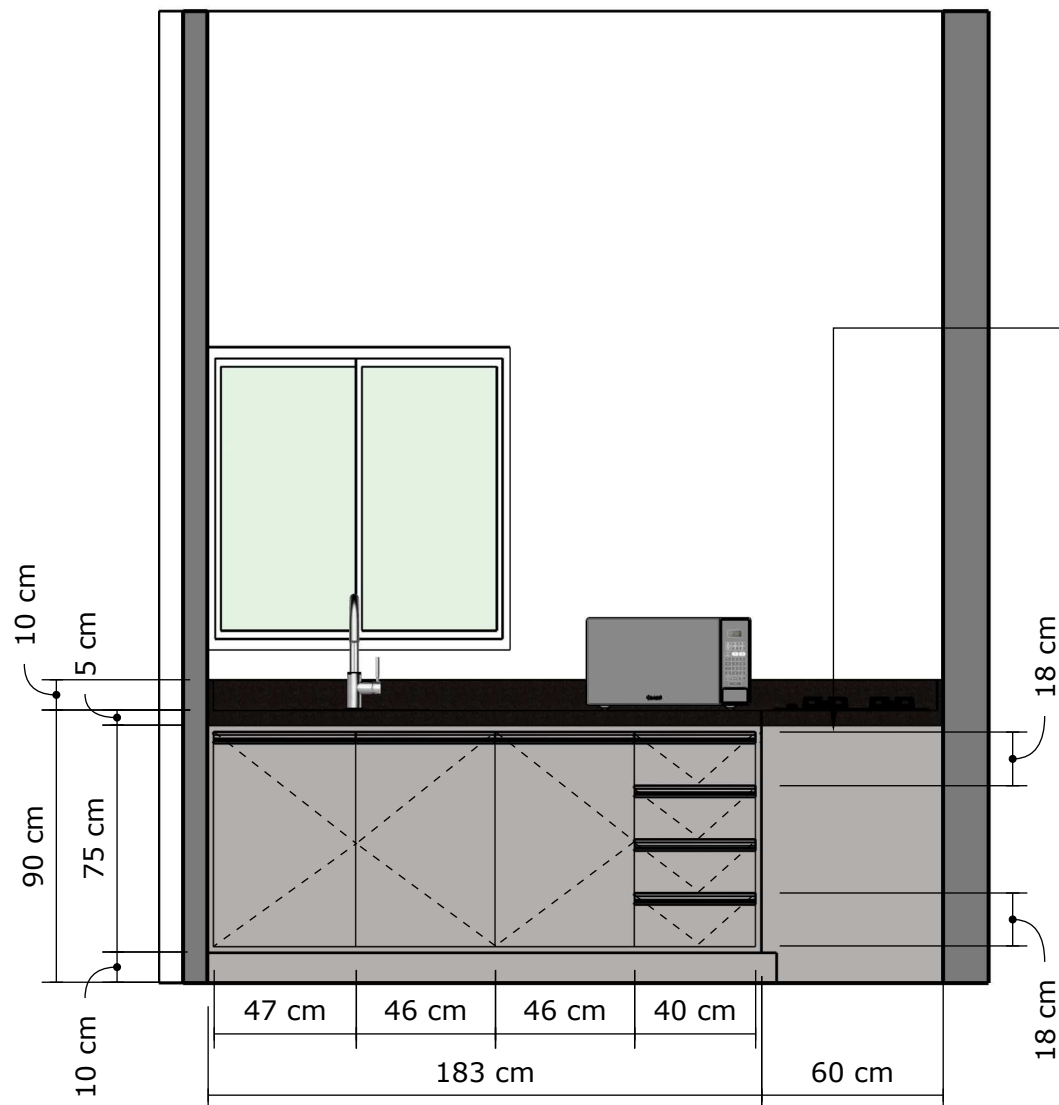
VISTA A
