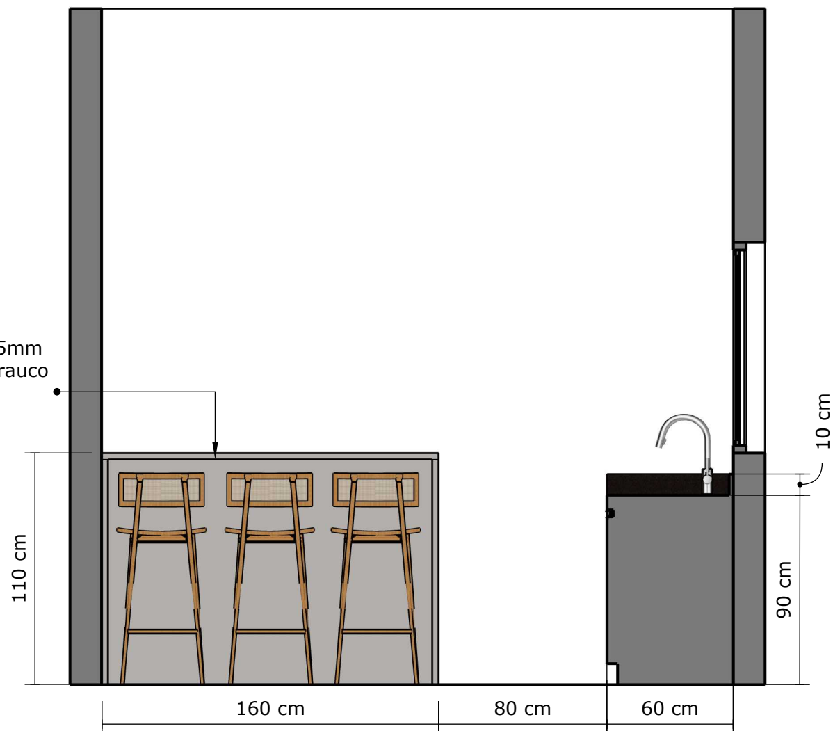
VISTA C
