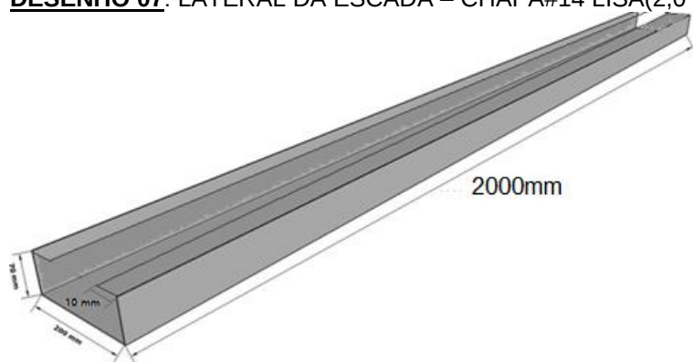
DESENHO 07 : LATERAL DA ESCADA – CHAPA#14 LISA(2,0 mm) – 32 PEÇAS
