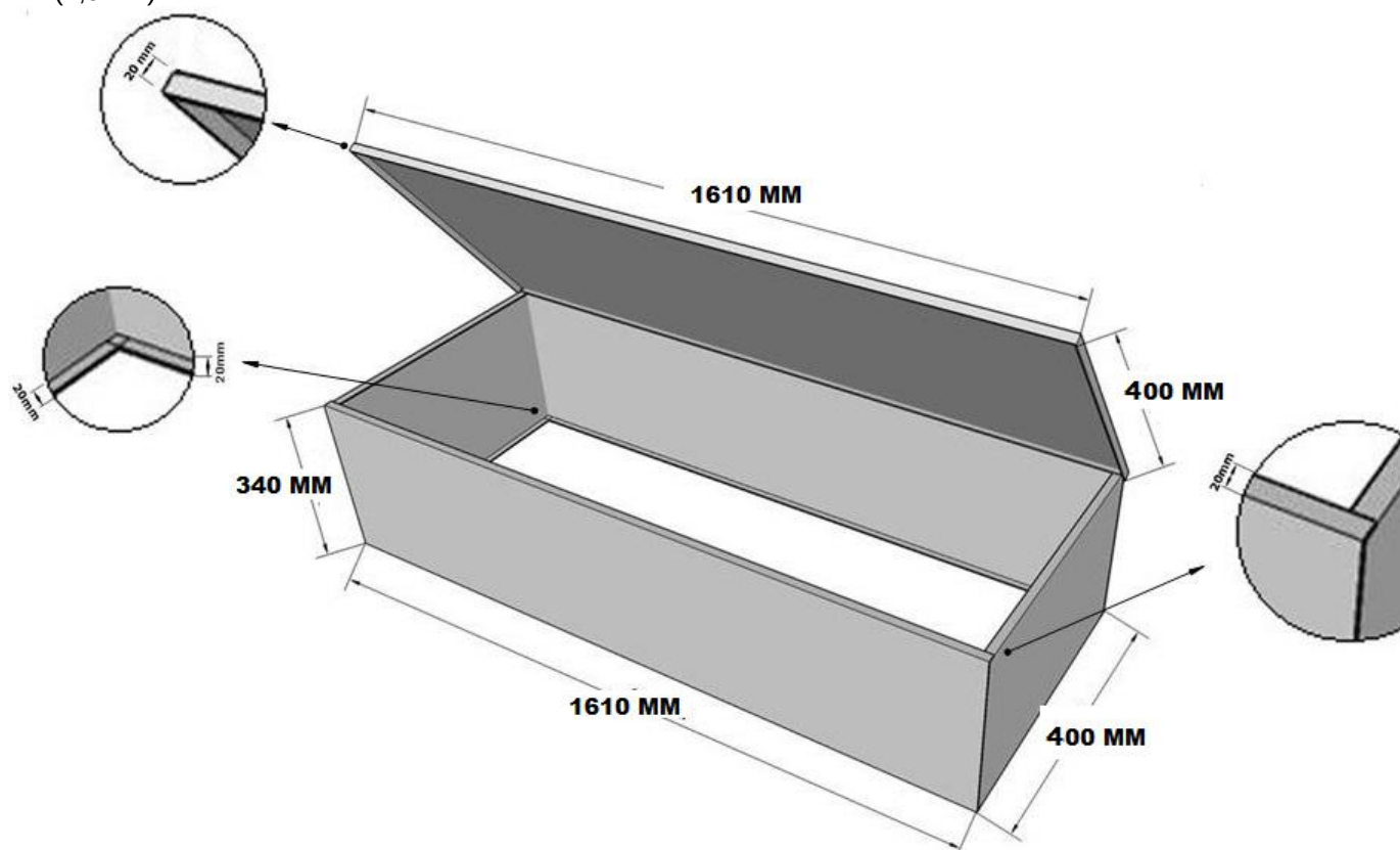
DESENHO 05-B: CAIXA DE PROTEÇÃO DOS MOTORES (VISTA MONTADA) – CHAPA #14(1,9mm)
