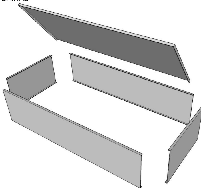
DESENHO 05-A: CAIXA DE PROTEÇÃO DOS MOTORES (VISTA EXPLODIDA) – CHAPA #14(1,9mm) – 80 CAIXAS
