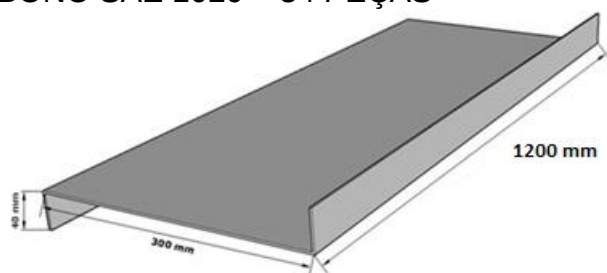
DESENHO 06: DEGRAU DA ESCADA – CHAPA AÇO XADREZ, 1/8" AÇO CARBONO SAE 1020 – 34 PEÇAS
