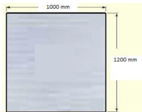
DESENHO 08 : PATAMAR ESCADA – 02 PEÇAS – CHAPA 1/8"
