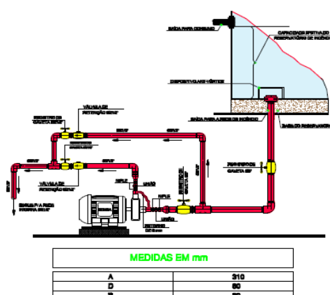
DETALHE DE BOMBA E RESERVA DE INCÊNDIO
