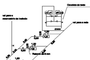
DETALHE DE BOMBA E RESERVA DE INCÊNDIO
