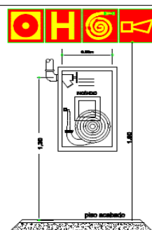
CAIXA DE HIDRANTES
