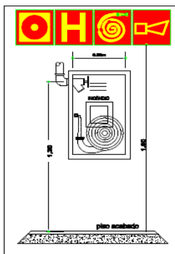
CAIXA DE HIDRANTES
