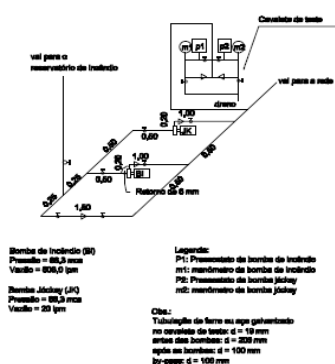
DETALHE DE BOMBA E RESERVA DE INCÊNDIO
