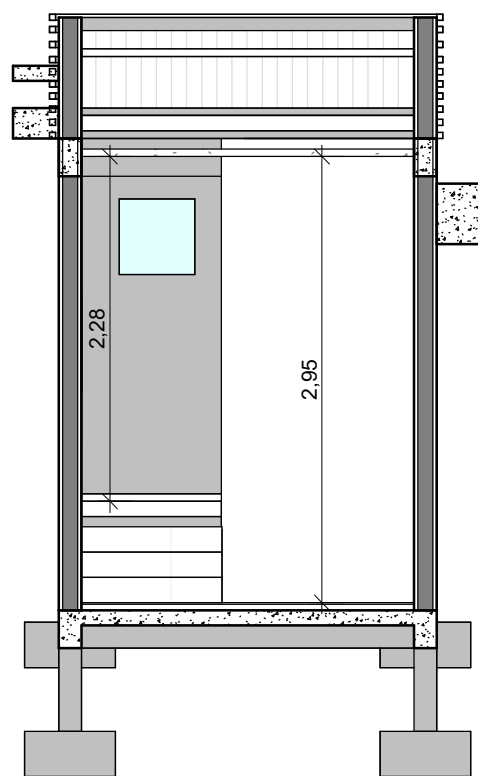
1 CORTE 01 ESCALA 1 : 50
