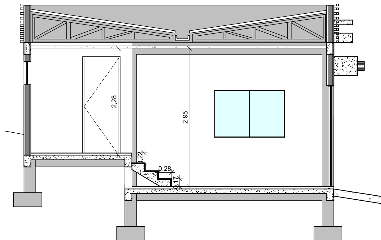
2 CORTE 02 ESCALA 1 : 50
