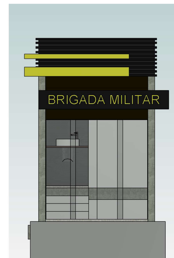
3 Fachada Frontal ESCALA 1 : 50
