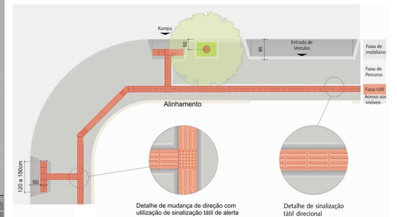
DETALHAMENTO | PISO TÁTIL E RAMPAS DE ACESSIBILIDADE
