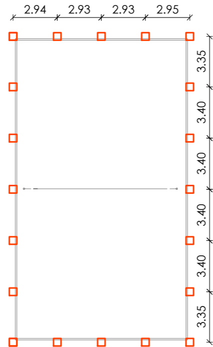
PLANTA BAIXA | quadra de areia PROJETO DE FUNDAÇÕES esc 1:250
