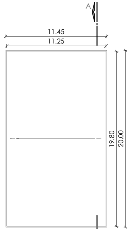
PLANTA BAIXA PROJETO EM AREIA esc 1:250 Área: 222,75m 2
