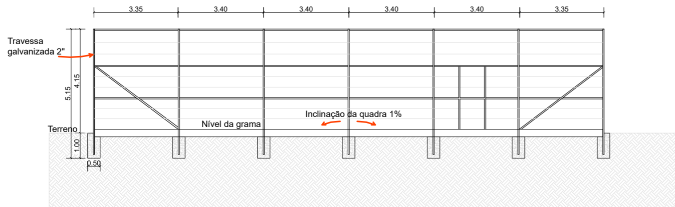
CORTE AA' - ALAMBRADO esc 1:150
