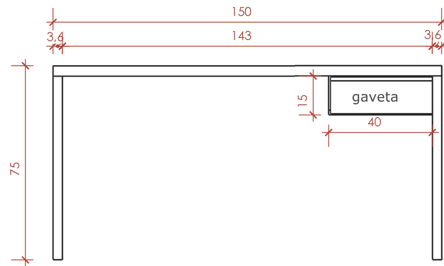
VISTA FRONTAL - CONSULTÓRIO ESC.: 1/15
