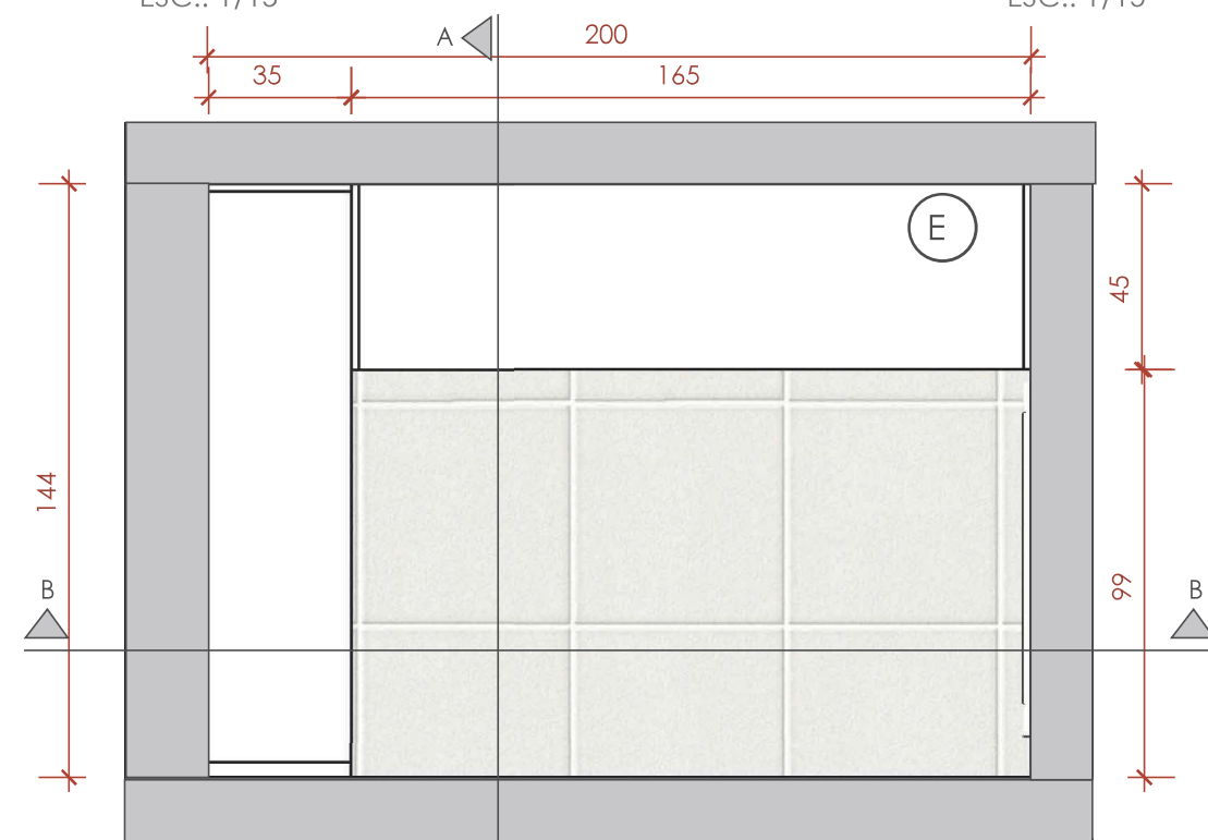
PLANTA- ESTOQUE
