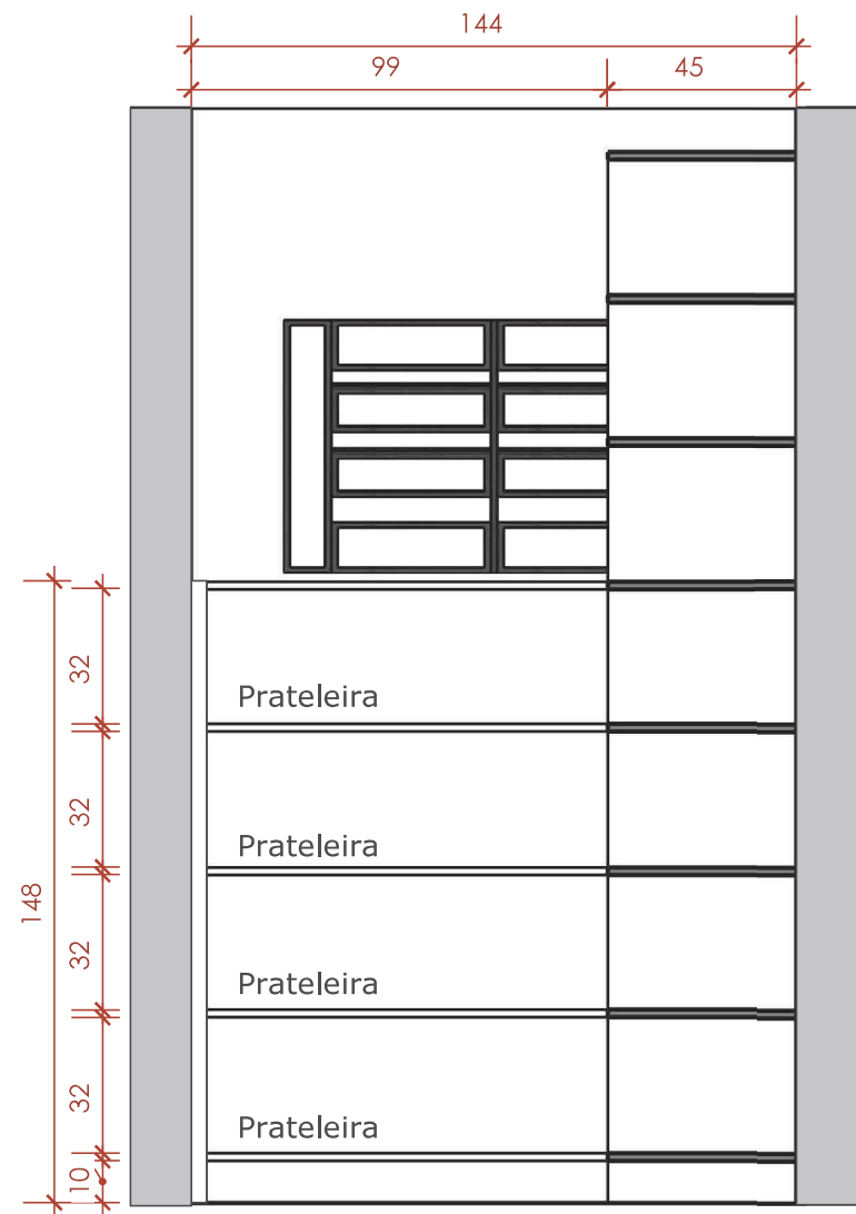
CORTE FRONTAL AA" - ESTOQUE
