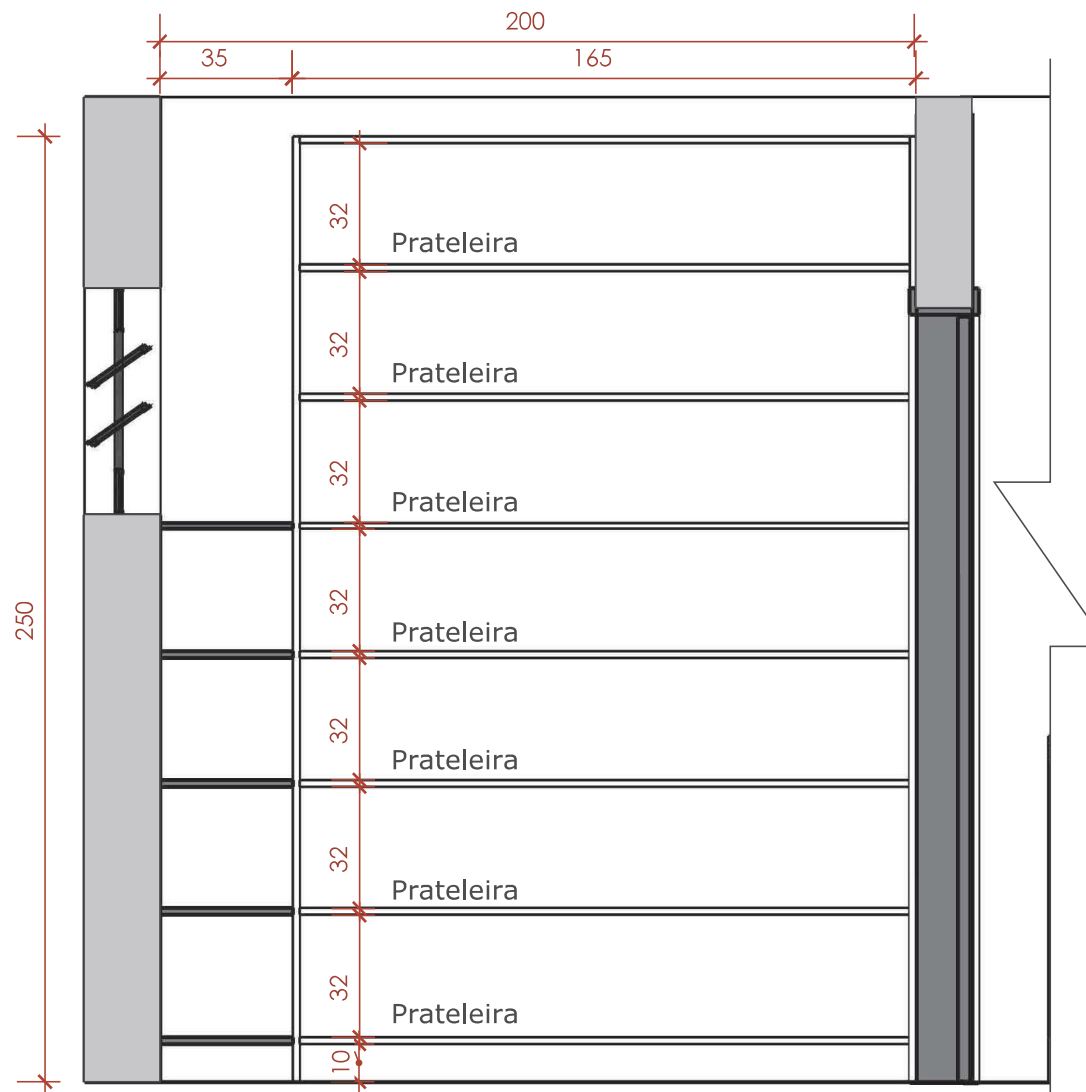
CORTE LATERAL BB" - ESTOQUE
